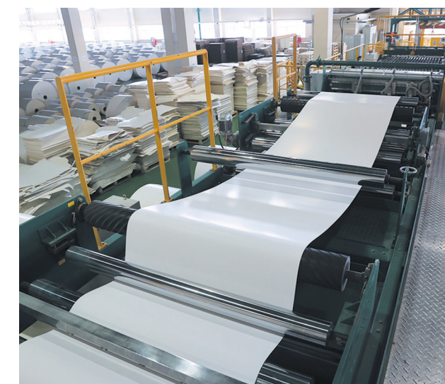
Участок форматной резки. Идет раскрой мелованного картона
